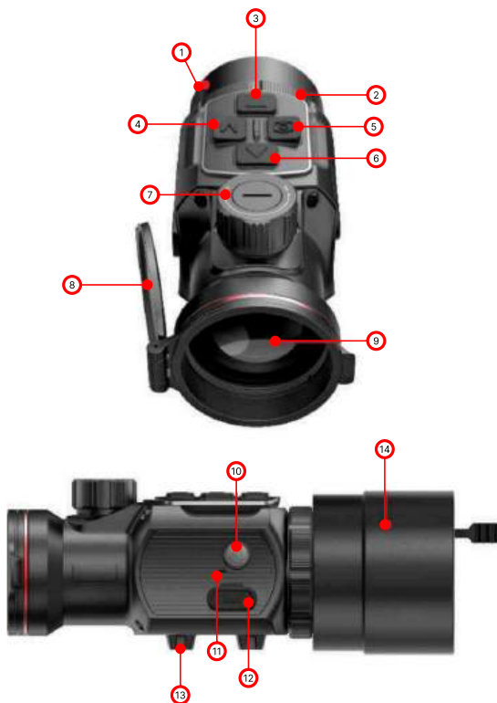
Рис. 1. Устройство тепловизионной насадки Longot Mate Y050 (МАН50)
