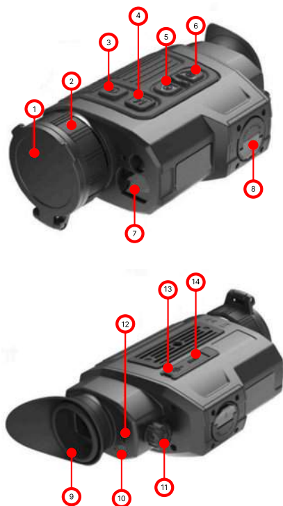
Рис. 1. Устройство тепловизионного монокуляра FH35R V2
