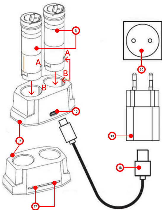
Рис. 3. Зарядка аккумуляторов в зарядном устройстве.
