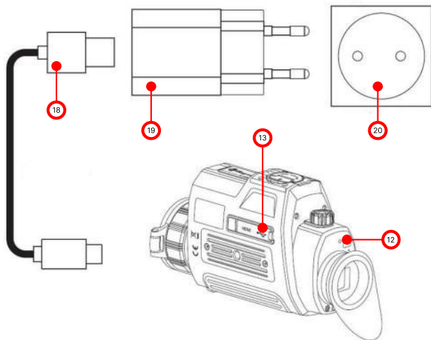
Рис. 2. Подключение прибора для зарядки от сети.
