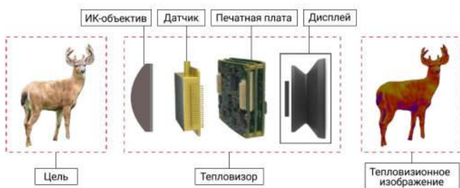
Рис. 1. Схема формирования изображения тепловизором.
